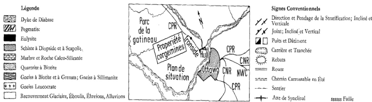
Fig. 2. Carte géologique et situation géographique de l'enveloppe du gisement de Forsyth
